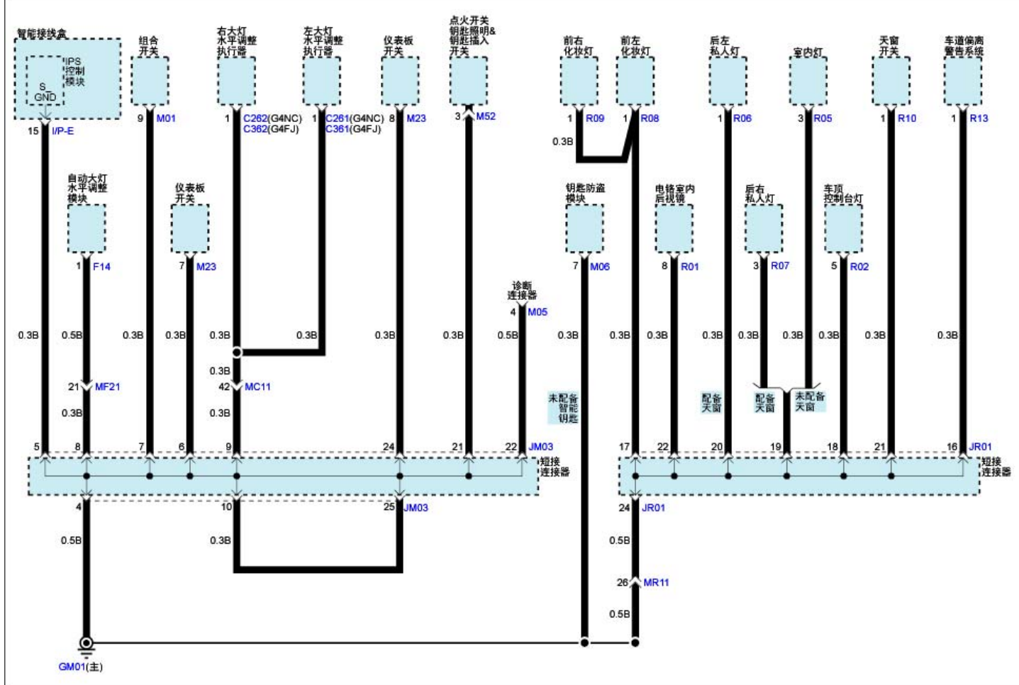
搭铁分布(1)
